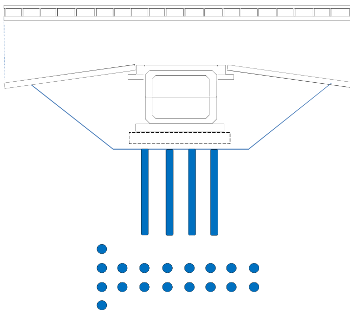
Obiekt 25 PZ km 461+124 istniejący
