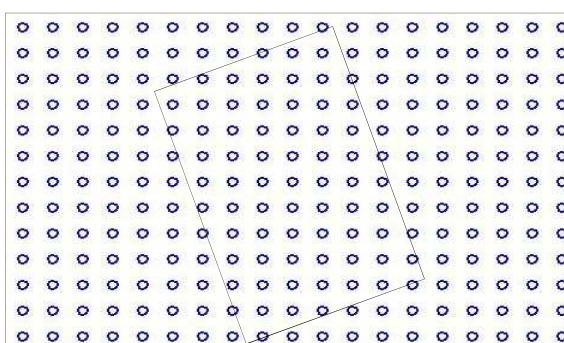
kontur obejmujący rozmieszczenie kolumn żwirowych
