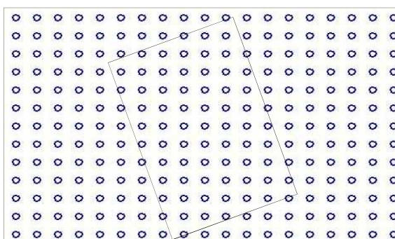
kontur obejmujący rozmieszczenie kolumn żwirowych
