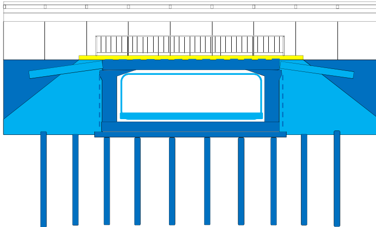
kontur obejmujący rozmieszczenie kolumn żwirowych
