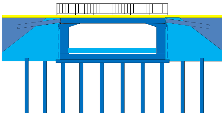
kontur obejmujący rozmieszczenie kolumn żwirowych
